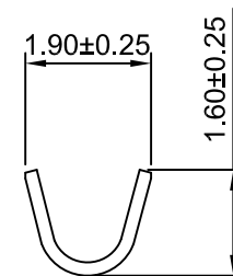
SEC:B-B
