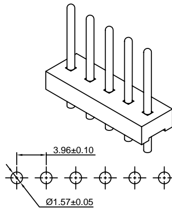
P.C.B LAYOUT
