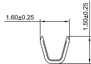
SEC:B-B
