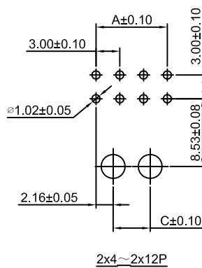
P.C.B LAYOUT
