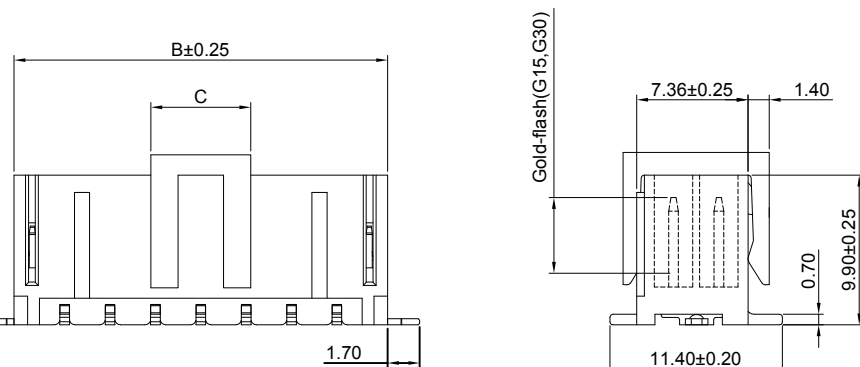
P.C.B LAYOUT
