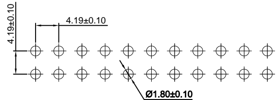
P.C.B LAYOUT
