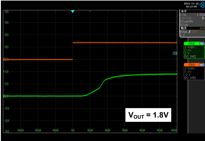
EN high
