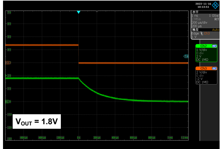
EN low
