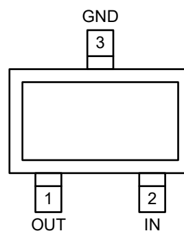
CJ6330AxxMY SOT-23-3L
