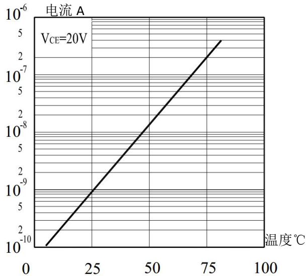
暗电流与温度的关系
