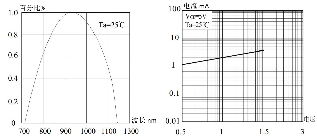
波长感应曲线图 集电极电流与电压关系
