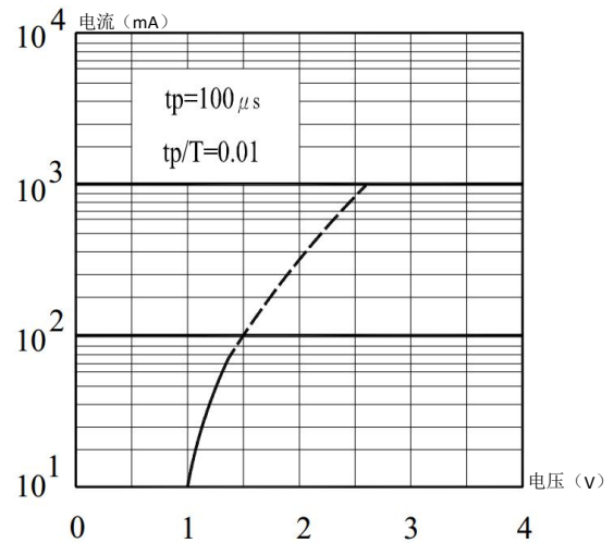
集电极电流与电压关系
