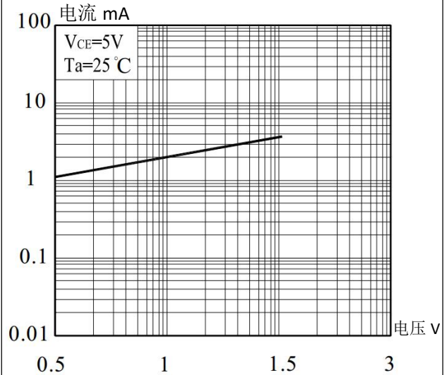
正向电流与正向电压的关系
