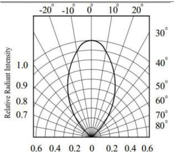
发射角度图
