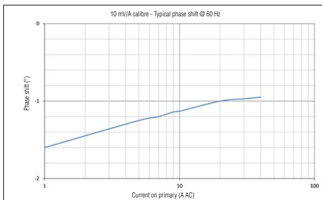
Phase shift
