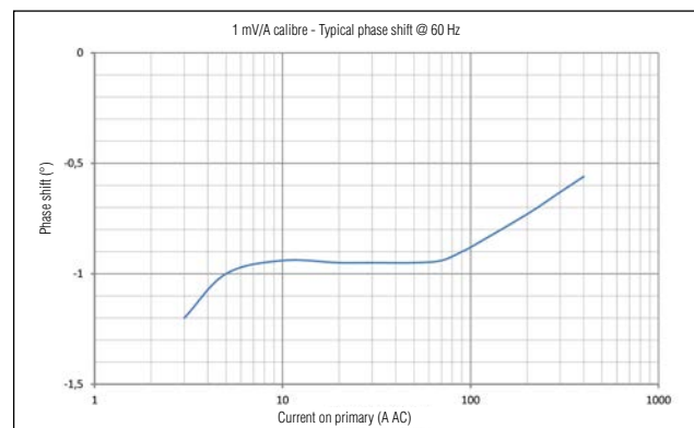
Phase shift
