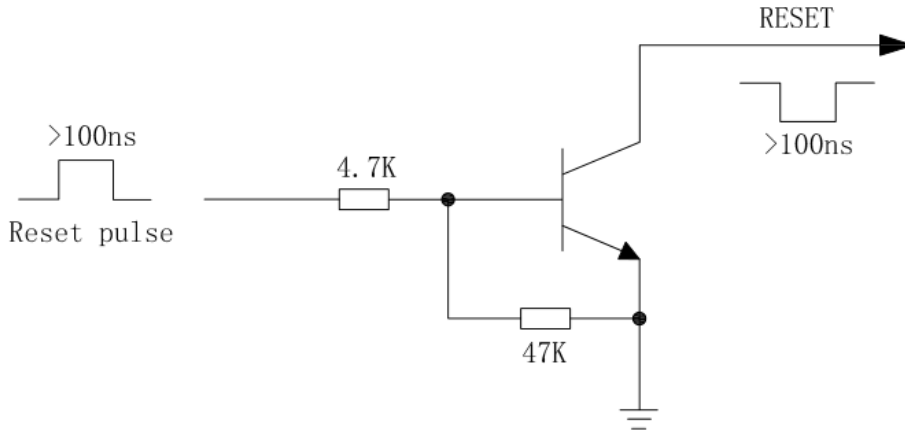
图 5 复位参考电路
