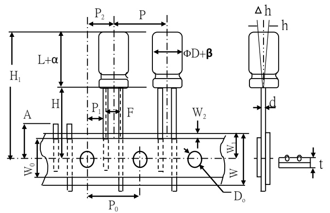
[ Fig. 4 (Diameter for \Phi 10 、 \Phi 13 、 \Phi 16 ) ]
