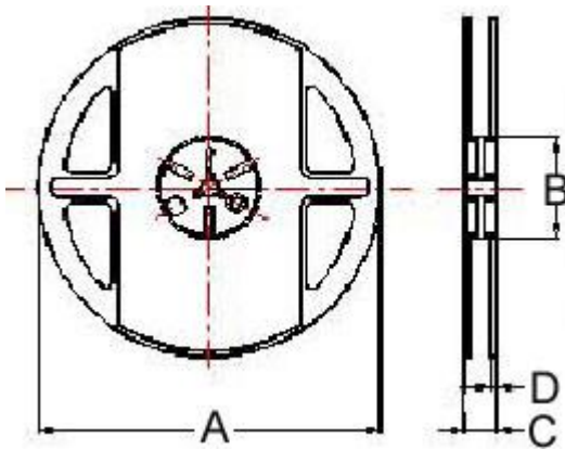
Reel Dimensions
