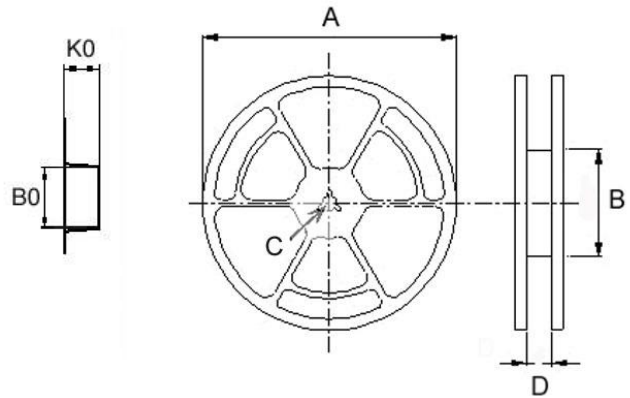
Reel Dimensions
