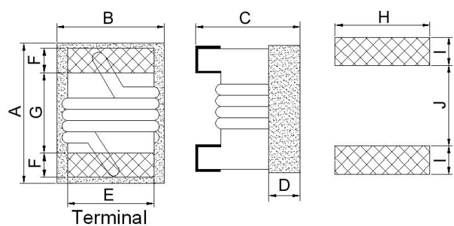
CS0402
