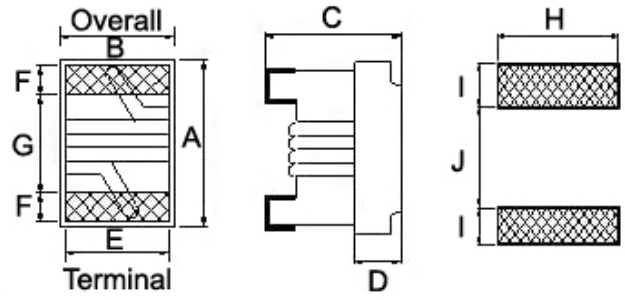
CM0603
