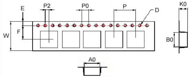
Reel Dimensions
