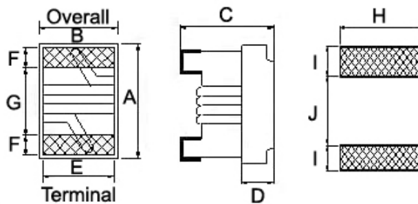
CM0603
