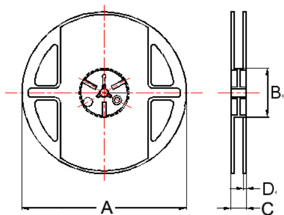
Reel Dimensions
