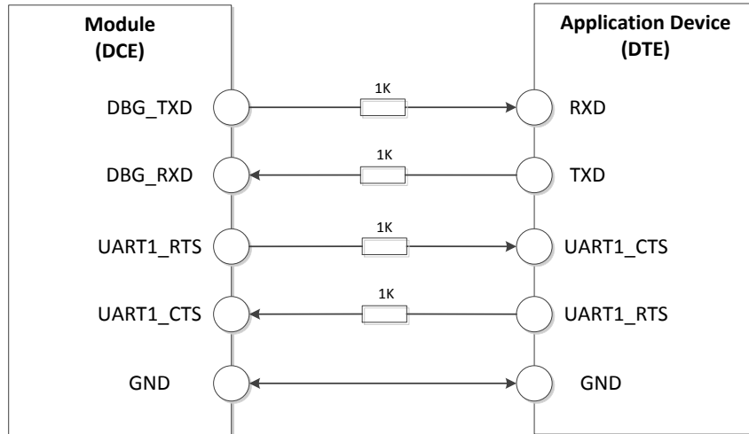
图 11: 1.8V 电平连接电路
