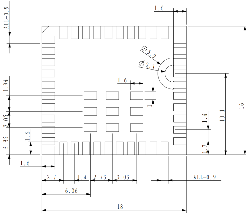
图 19: M5311 机械尺寸图 (Top View, 单位: 毫米)
