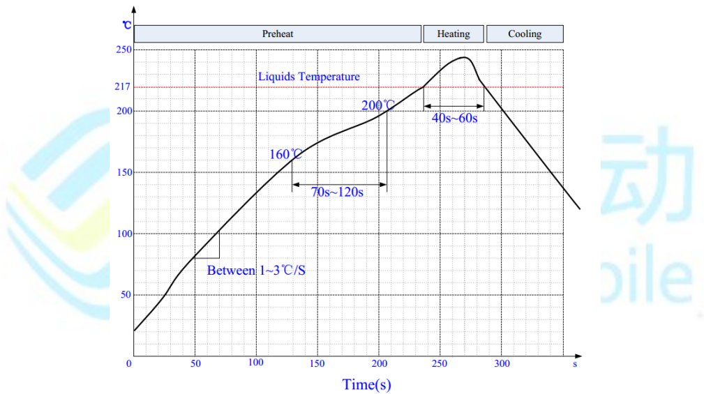
图 24: 炉温曲线
