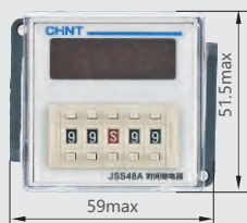
JSS48A系列产品外形及安装尺寸
