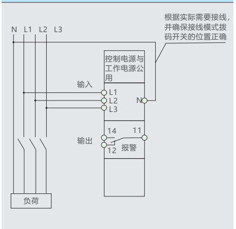
接线图
