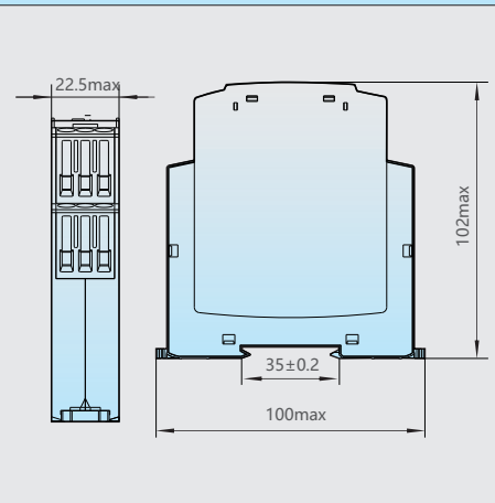
外形尺寸
