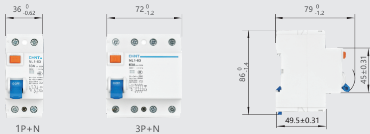
图1 外形及安装尺寸
