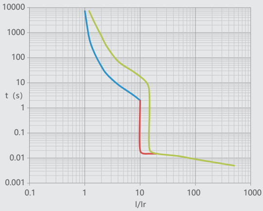
图23 NM1-250电动机保护
