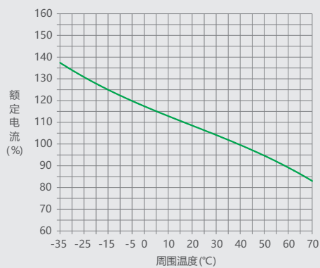
图20 NM1-125 63A以上 温度补偿曲线
