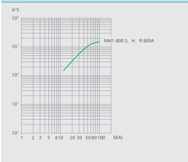
图43 NM1-800 允通曲线
