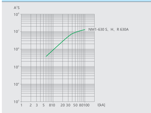
图42 NM1-630 允通曲线
