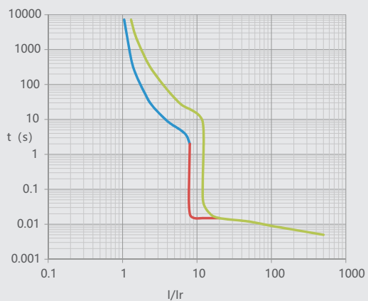
图19 NM1-125 63A以上电动机保护
