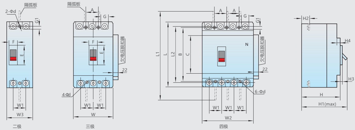
NM1-63、125、250外形及安装尺寸(板前接线)(见表8)
