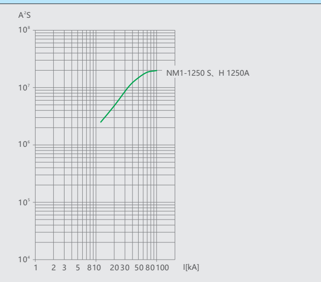
图44 NM1-1250 允通曲线
