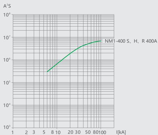
图41 NM1-400 允通曲线
