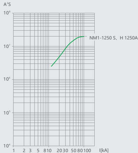
图44 NM1-1250 允通曲线
