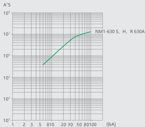
图42 NM1-630 允通曲线
