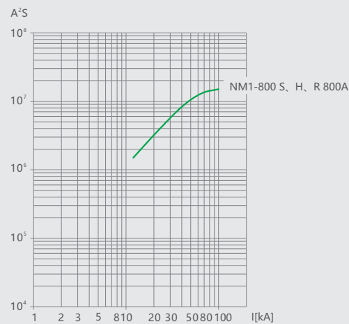
图43 NM1-800 允通曲线
