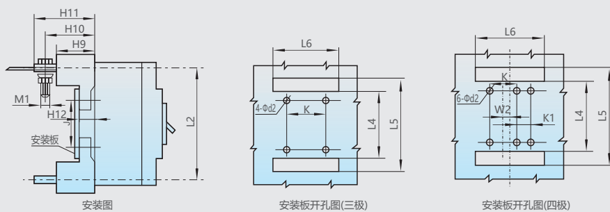
安装图
