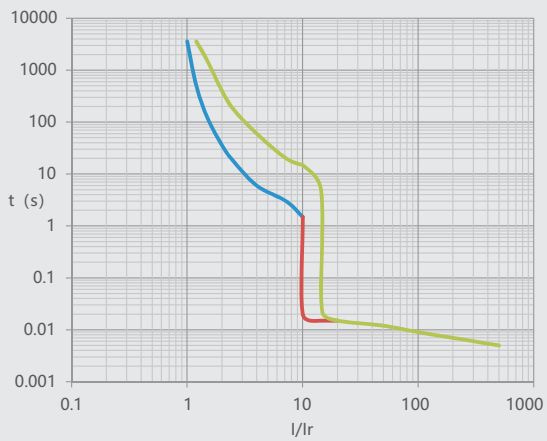
图3 NM1LE-125 16A~25A电动机保护
