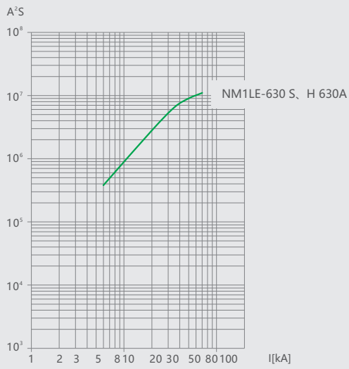
图5 NM1LE-630 允通曲线
