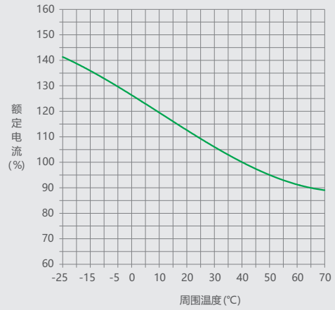
图22 NM1LE-630 温度补偿曲线
