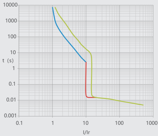
图27 NM1LE-800电动机保护
