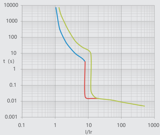
图13 NM1LE-250 配电保护
