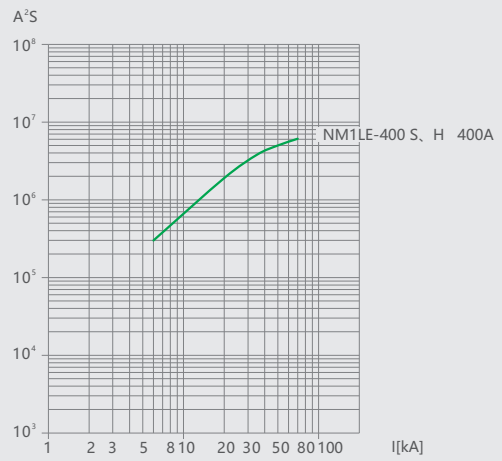
图4 NM1LE-400 允通曲线
