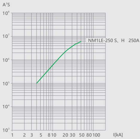
图3 NM1LE-250 允通曲线
