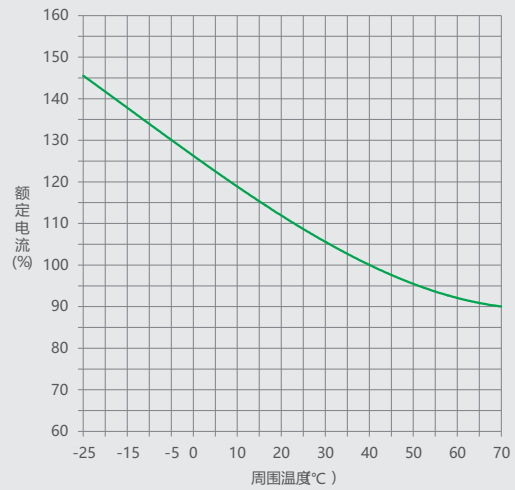
图28 NM1LE-800 温度补偿曲线
