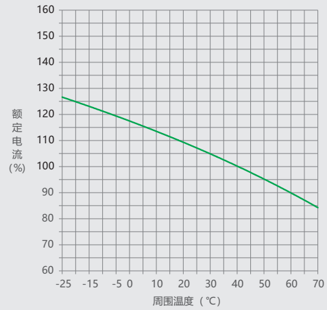
图16 NM1LE-250 温度补偿曲线
