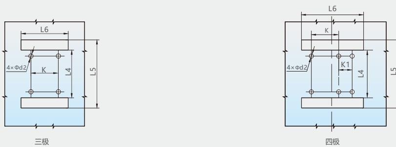
插入式接线开孔图(尺寸见表14)
