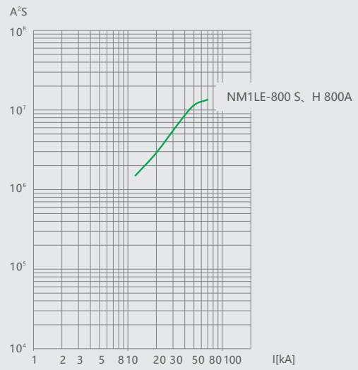
图6 NM1LE-800 允通曲线
