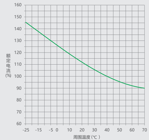
图26 NM1LE-800 温度补偿曲线
