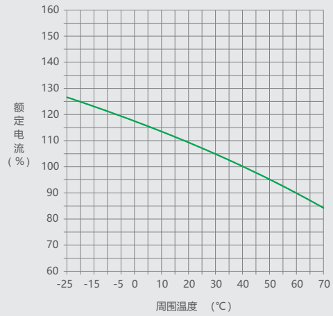
图6 NM1LE-125 32A-63A 温度补偿曲线
