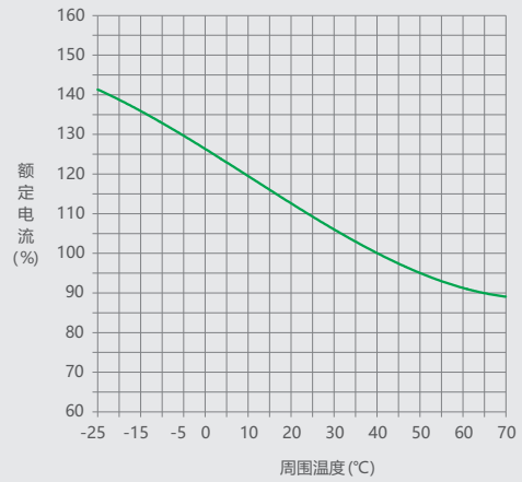
图26 NM1LE-800 温度补偿曲线
