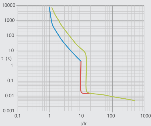
图19 NM1LE-400 电动机保护
