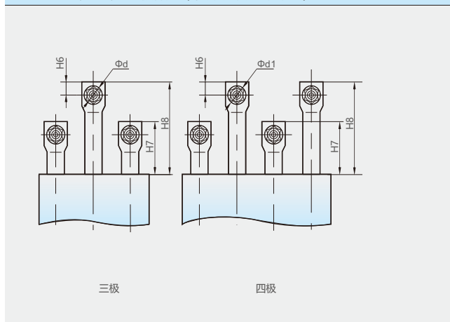
NM1LE-400, 630, 800板后接线(外形及安装尺寸见表14)
