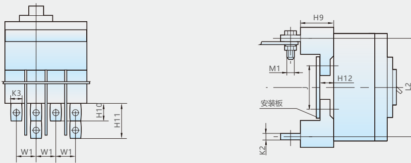
插入式接线图(安装尺寸见表14)
