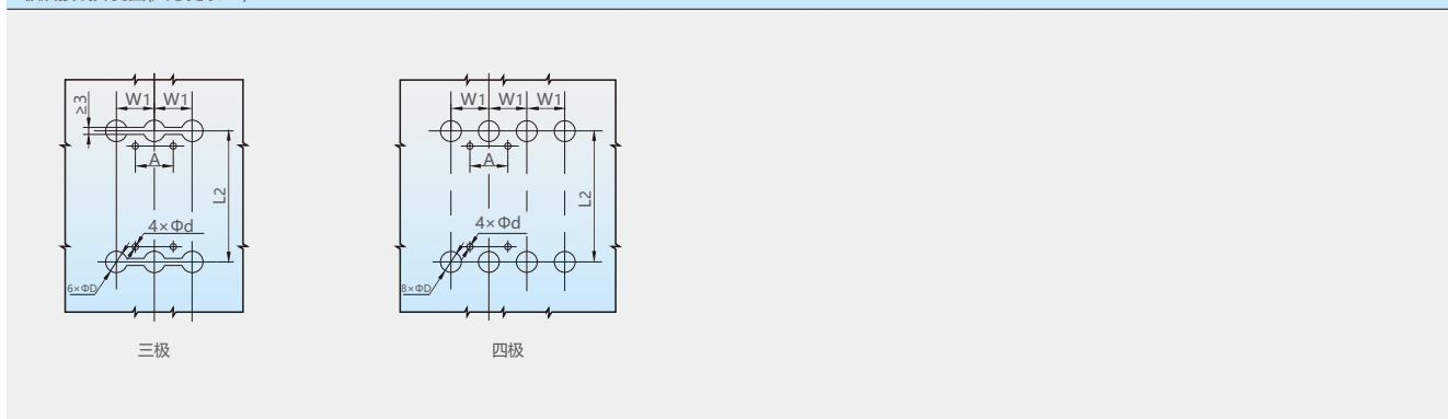
板后接线开孔图(尺寸见表14)
