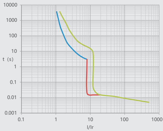
图5 NM1LE-125 32A-63A 配电保护
