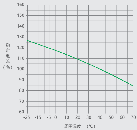
图8 NM1LE-125 32A-63A 温度补偿曲线
