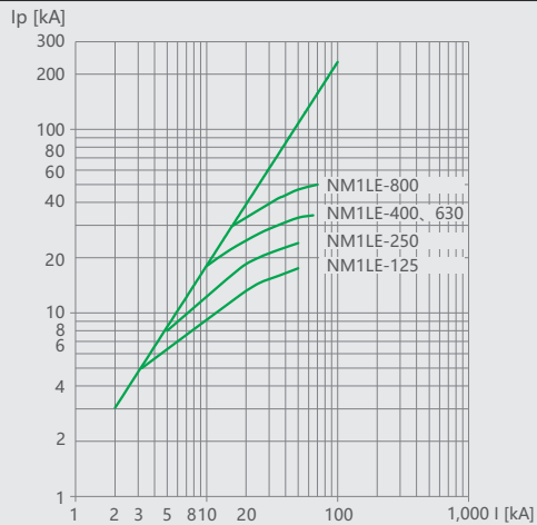
图1 AC400V/415V的NM1LE系列限流曲线图
