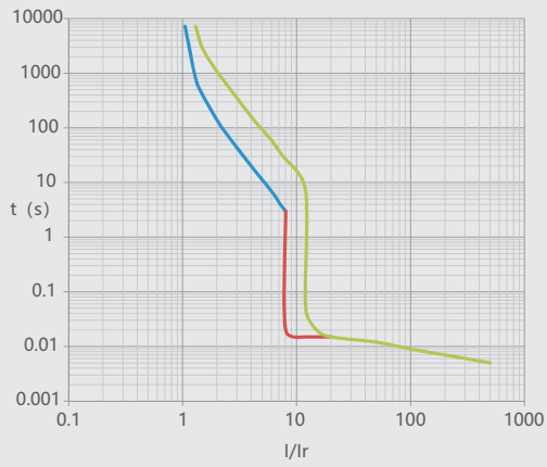
图21 NM1LE-630 配电保护
