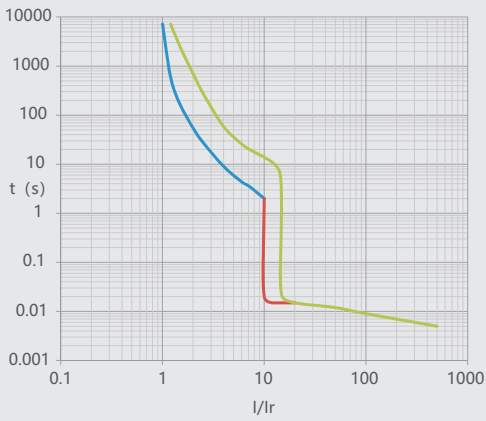
图15 NM1LE-250 电动机保护
