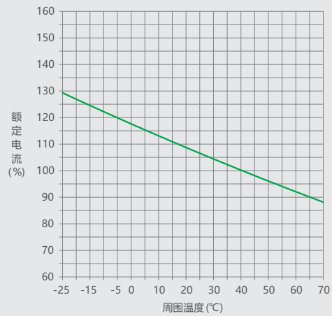
图18 NM1LE-400 温度补偿曲线
