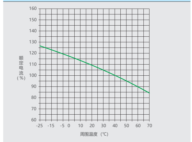
图2 NM1LE-125 16A-25A 温度补偿曲线
