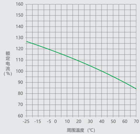
图4 NM1LE-125 16A-25A 温度补偿曲线
