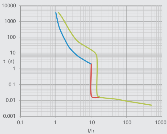
图7 NM1LE-125 32A-63A 电动机保护
