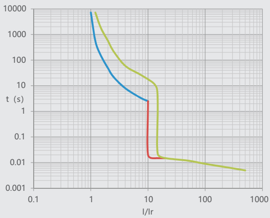
图11 NM1LE-125 >63A 电动机保护
