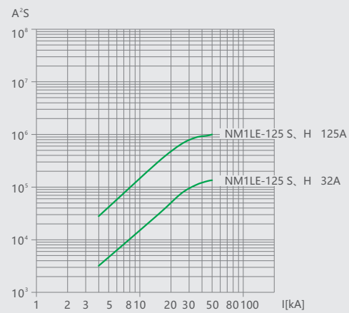
图2 NM1LE-125 允通曲线
