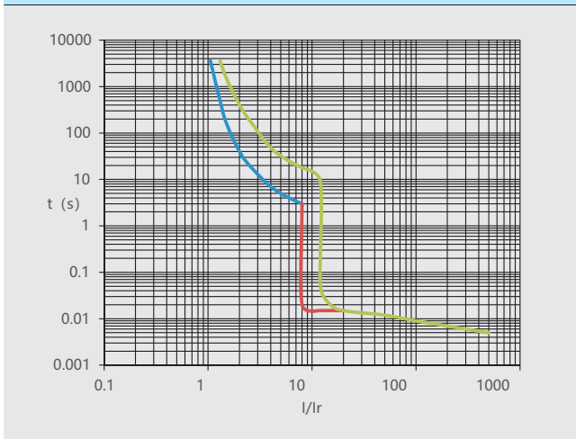
图1 NM1LE-125 16A~25A配电保护
