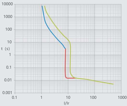
图17 NM1LE-400 配电保护
