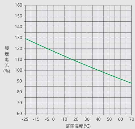
图20 NM1LE-400 温度补偿曲线
