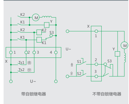
NM1LE-400电动机接线图
