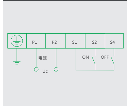
NM1LE-125、250、400、630、800电动机接线图
