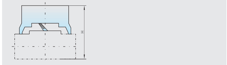
电动操作机构安装尺寸图
