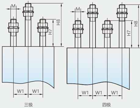
板后接线开孔图(尺寸见表14)
