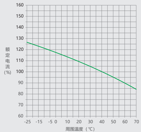
图14 NM1LE-250 温度补偿曲线
