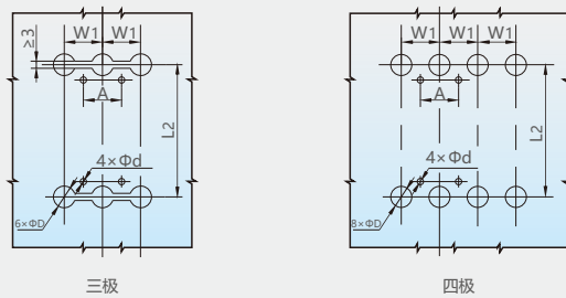
板后接线开孔图(尺寸见表14)
