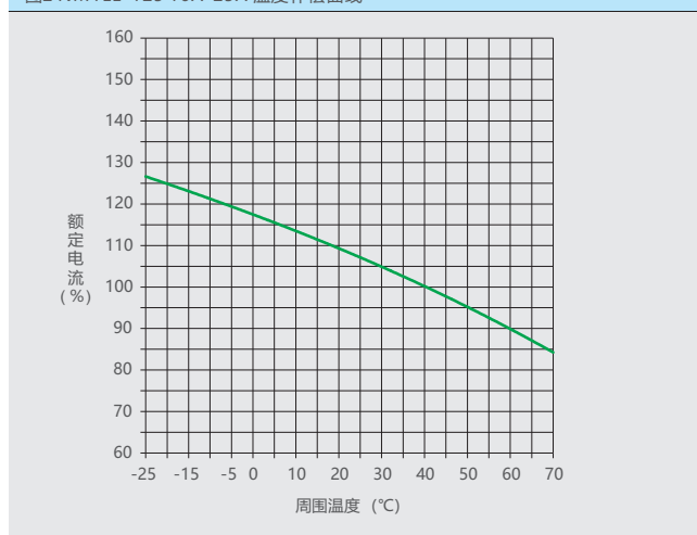
图2 NM1LE-125 16A-25A 温度补偿曲线
