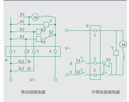
NM1LE-400电动机接线图
