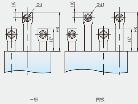
NM1LE-400, 630, 800板后接线(外形及安装尺寸见表14)
