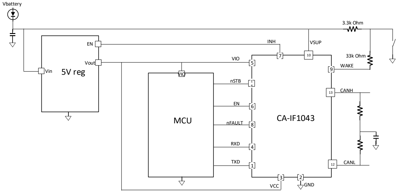
图 10-1 CA-IF1043 CAN 总线与 5V 稳压器的典型应用图
