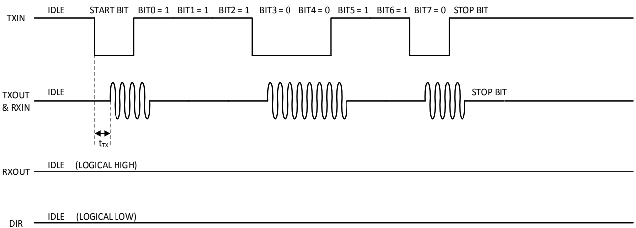
图 9-2 通信信号从 TXIN 传输到 TXOUT 的时序图
