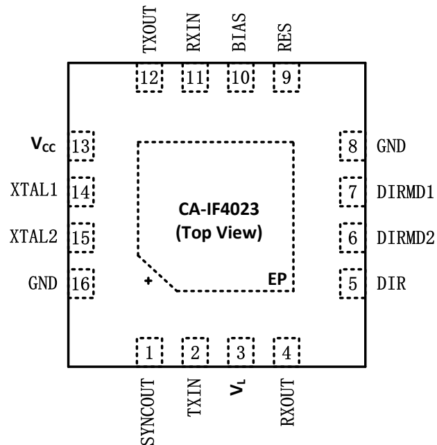
图 6-1 CA-IF4023 引脚图
