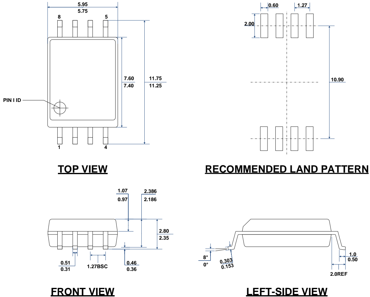
图 10-1 SOIC8 宽体封装外形尺寸图
