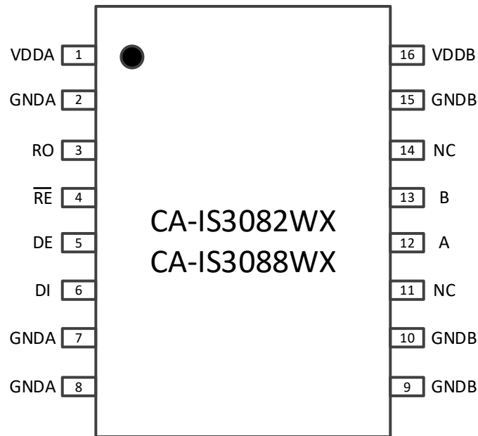
图 6-2 CA-IS3082WX 和 CA-IS3088WX 顶部视图
