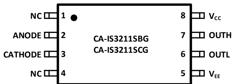
图 6-2 CA-IS3211SBG/ CA-IS3211SCG SOIC8-WB 配置
