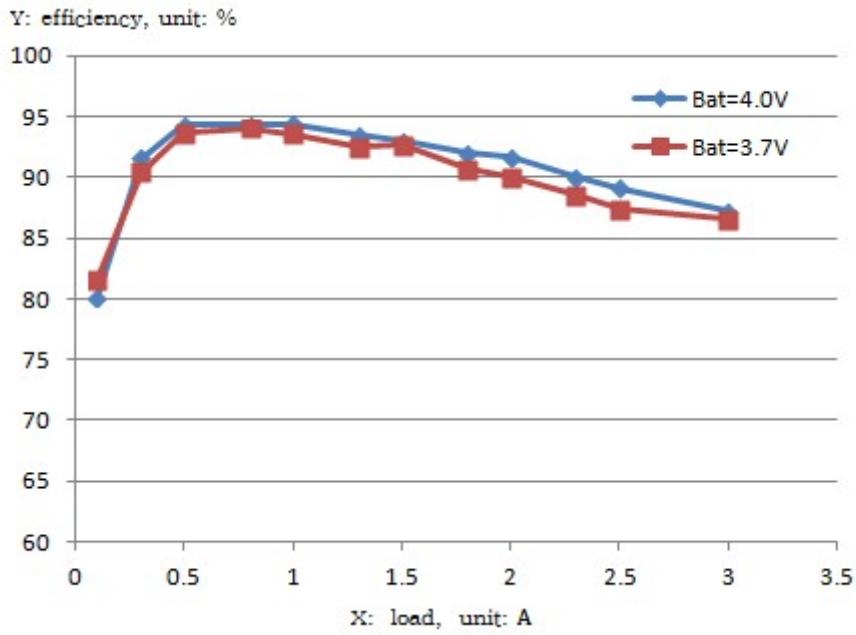
图 5 放电时效率与负载及 BAT 电压曲线
