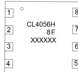
DFN3*3-8L
