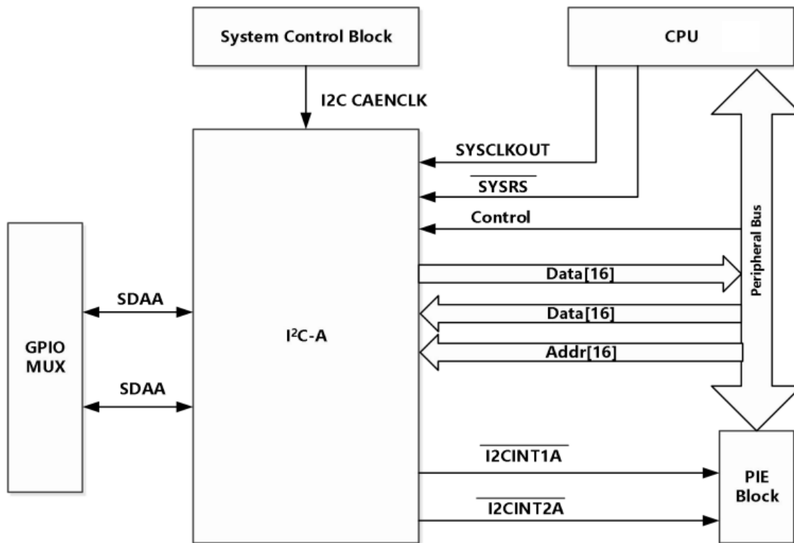
I2C 外设模块接口
