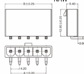
● Wafer XD-5557-NAW
