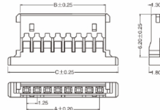
XD-CB1.25-NY
