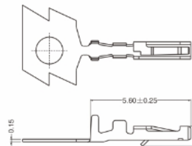
XD-CB1.25-NT
