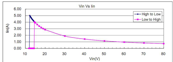
CQB50W12-72SXX-CMFC(D) Iin Vs Vin
