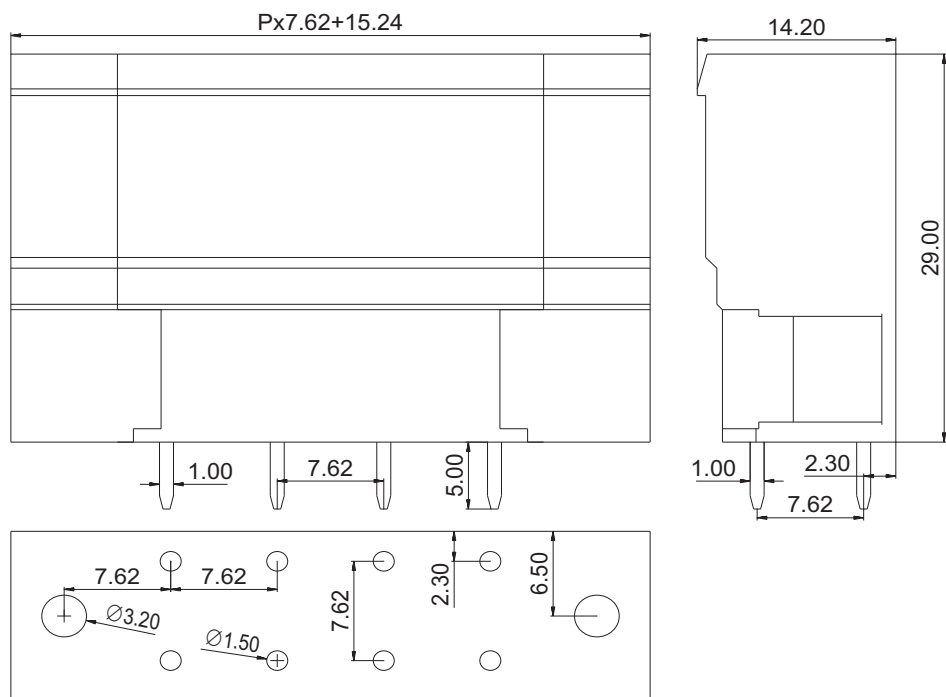
KF2EDGSVM-7.62
