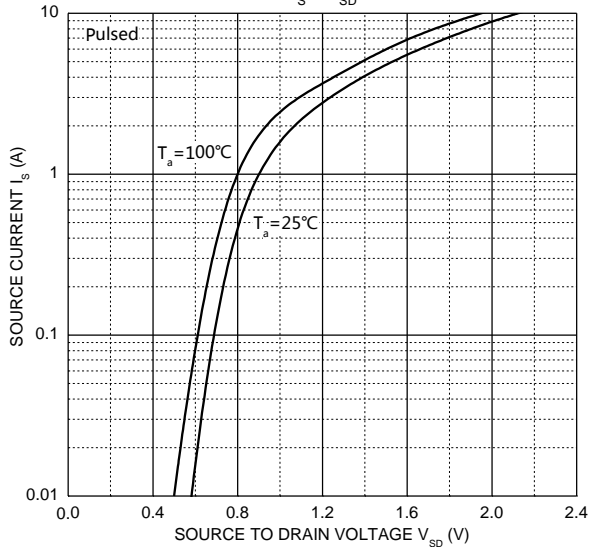
I_S - V_{SD}
