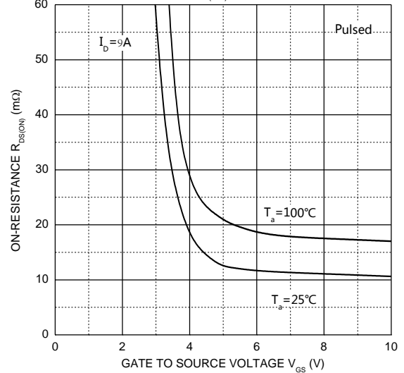
R_{DS(ON)} - V_{GS}
