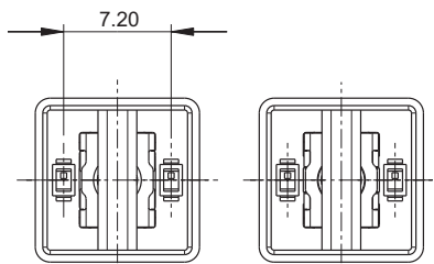
Stößel / plunger □ 11 mm
