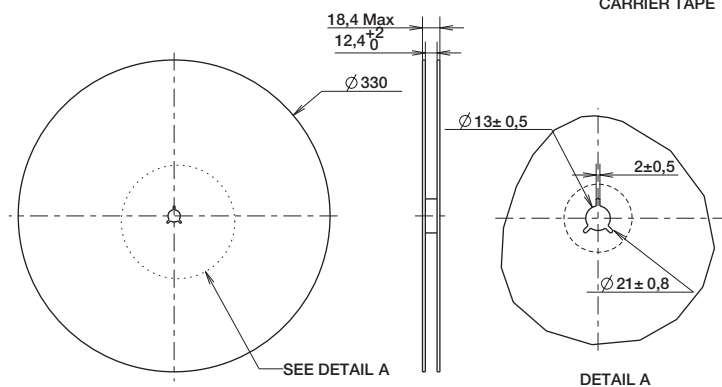
DETAIL A SCALE 0,5
